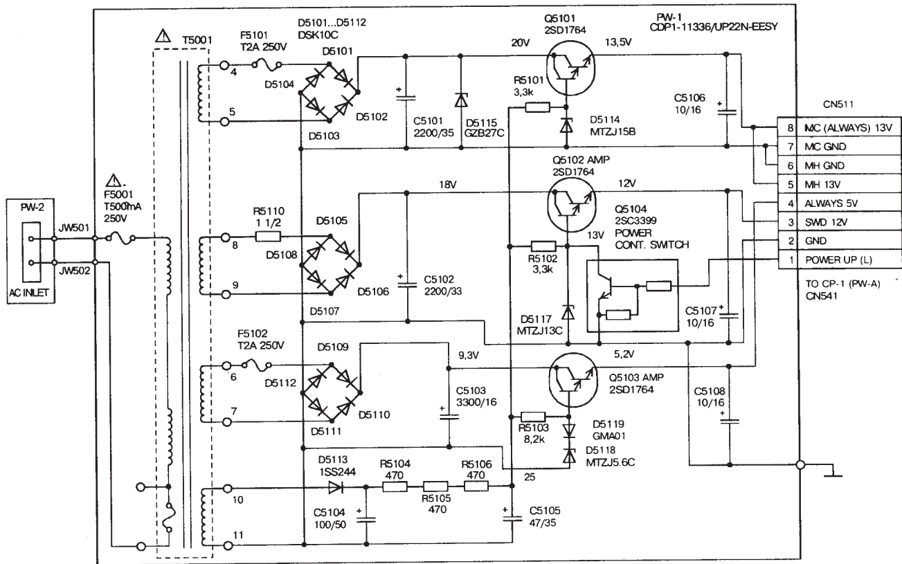
Принципиальная схема источника питания видеомагнитофона SLV-P116EE фирмы SONY.
