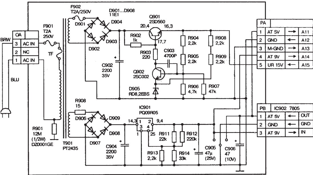
Принципиальная схема источника питания видеомассетопроигрывателя VC-6V3DR фирмы SHARP.
