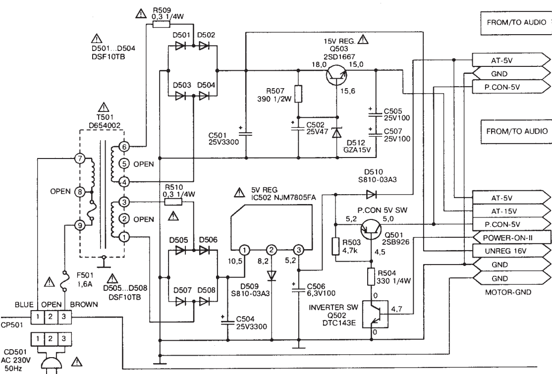
Принципиальная схема источника питания видеоплейеров ORION-388, ОТАКЕ V-33.
